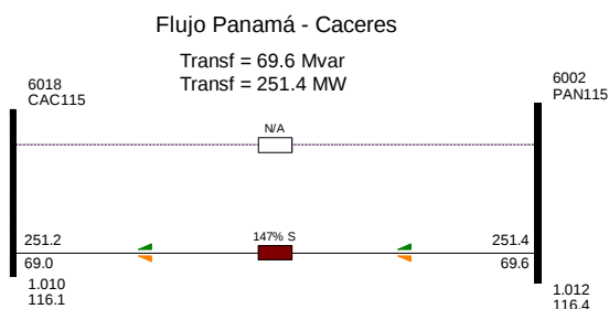
Figura 7. 1 Flujo línea 115-37 - falla 115-12, Sin Generación en Zona Atlántica
