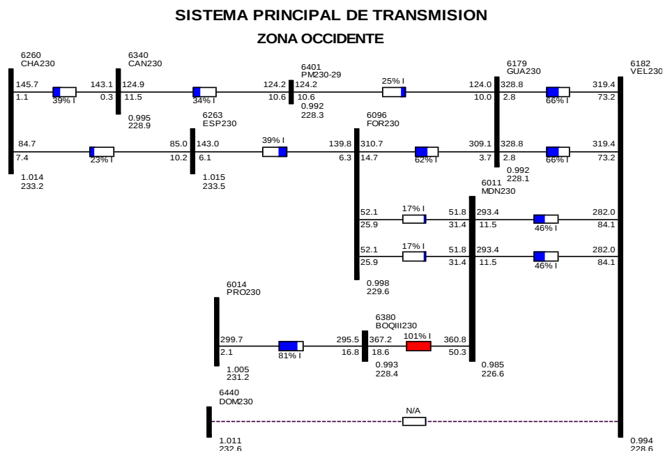
Figura 7. 8 Flujo línea 230-9a - falla 230-25a, Generación Total de la Zona
