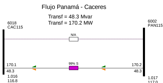
Figura 7. 2 Flujo línea 115-37 - falla 115-12, Con Generación en Zona Atlántica.
